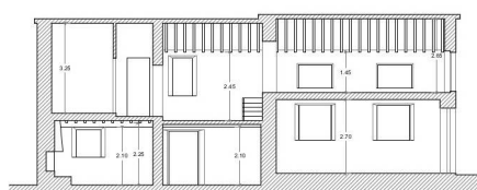
SEZIONE C - C'
